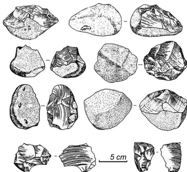
Рис. 1. Орудия эпохи олдувая, по: [14]. Fig. 1. Tools of the Oldowan period, according to: [14].
