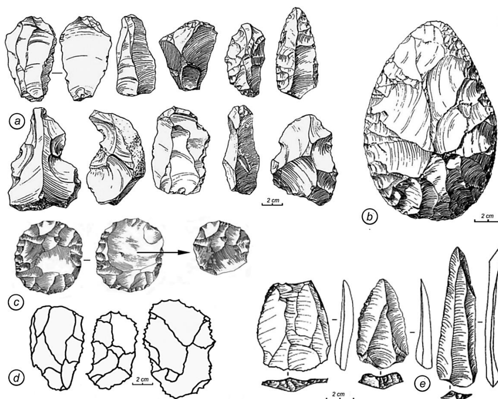
Рис. 4. Орудия ашельской культуры (а); ашельский бифас (b); пренуклеус, нуклеус и финальный отщеп в процессе леваллуа (с); абрис типичных черепаховидных снятий леваллуа из экспозиции Музея доистории (Лез-Эзи-де-Тайак-Сирёй, Франция) (d); мустьерские снятия из IX слоя пещеры Табун (е), по: [25; 26]
